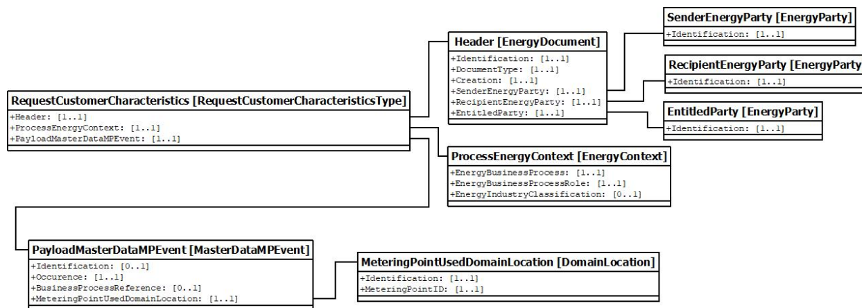
Slika 7: Dijagram klase za XML šemu RequestCustomerCharacteristics
