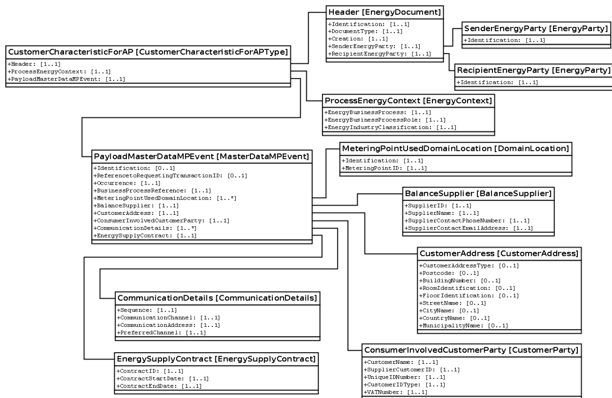
Slika 8: Dijagram klase za XML šemu CustomerCharacteristicsForAP
